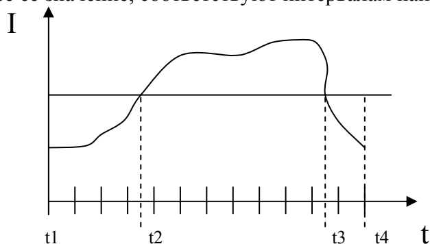
Рисунок А1. Типовой суточный график нагрузки центра питания
