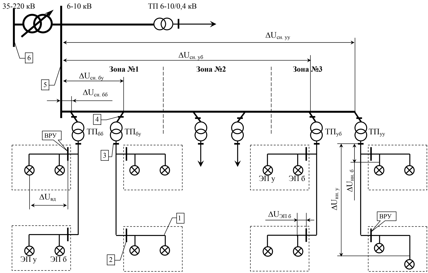
Рисунок А2 Схема распределительной электрической сети
