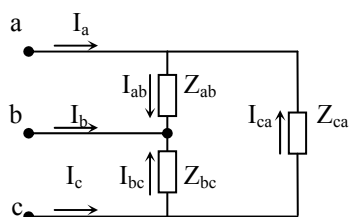
Рисунок Б.6 – Схемы соединения нагрузок ТН треугольником для трехпроводной измерительной цепи.
