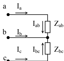
Рисунок Б.5 – Схема соединения нагрузок ТН открытым треугольником для трехпроводной измерительной цепи.
