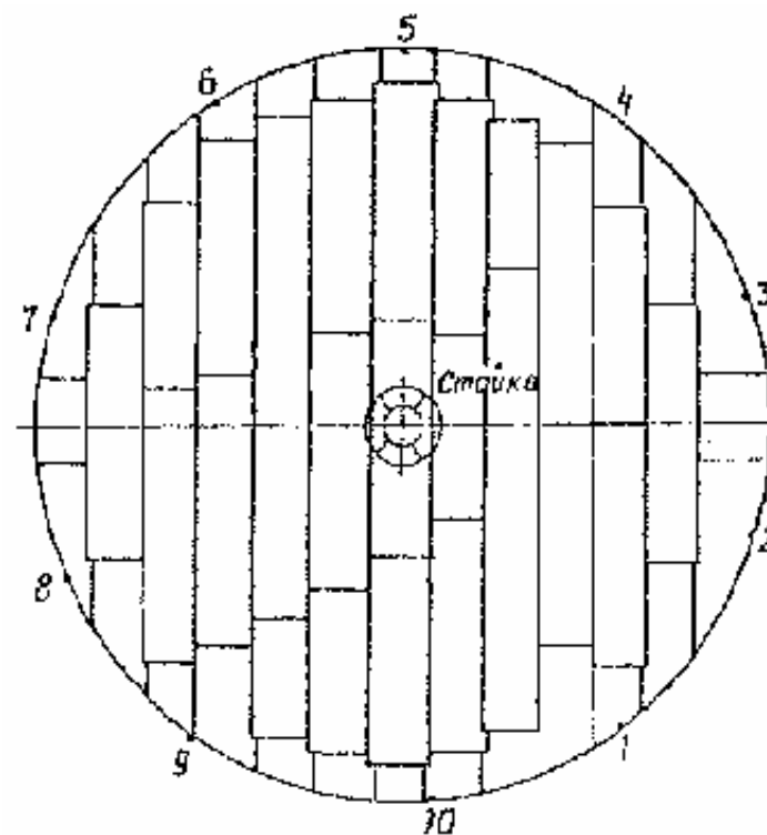
Рис. 4. Пример карт для обследования дна бака
