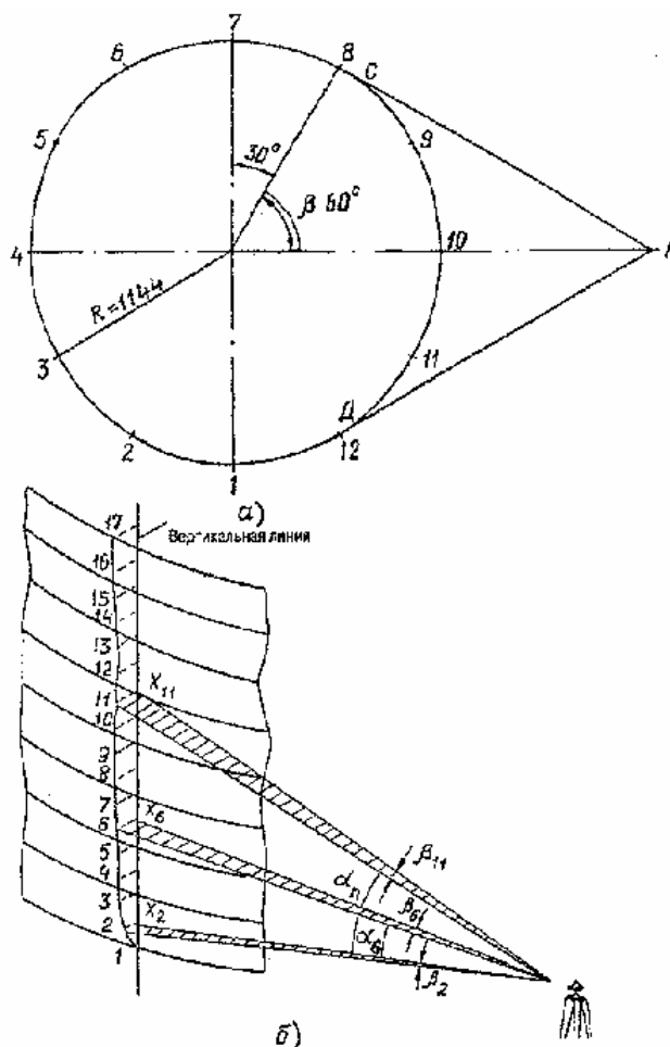
Рис.9. Определение отклонений стенки бака от вертикали с помощью теодолита: а - определение места (точка А) для установки теодолита; б - измерение горизонтальных и вертикальных углов
