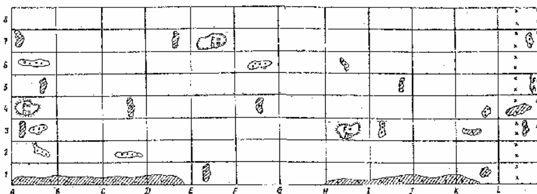
Рис. 7. Пример карты дефектов стенки баков
