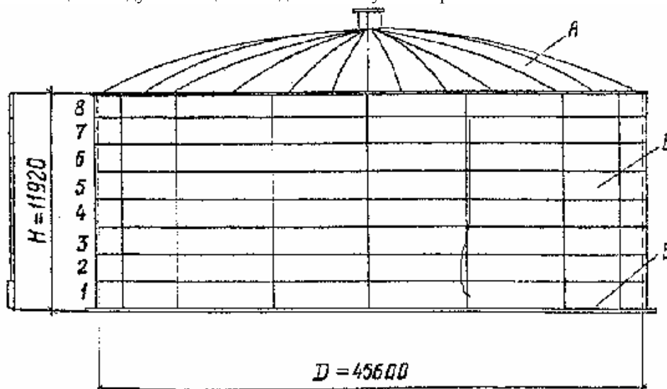
Рис. 1. Общий вид бака-аккумулятора вместимостью 20 тыс.м 3 : А - кровля; Б - стенка; В - днище
