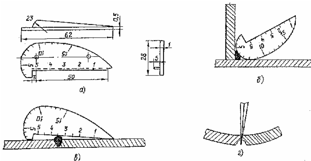
Рис.6. Шаблон для измерения габаритных размеров сварных соединений: а - общий вид шаблона; б - измерение высоты углового шва; в - измерение высоты стыкового шва; г - измерение зазора
