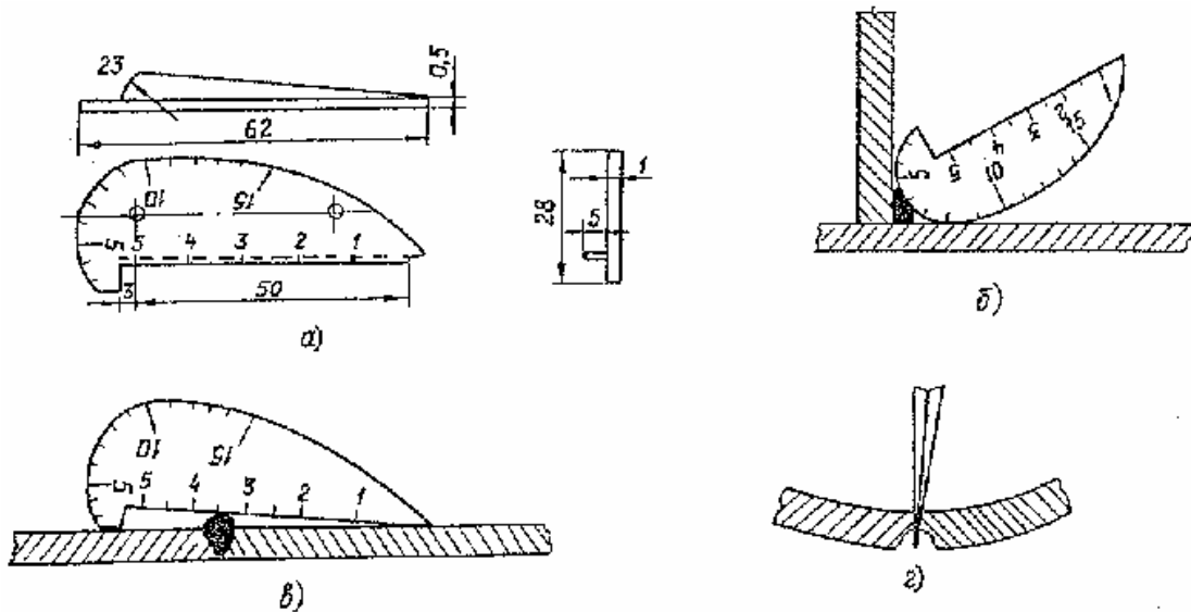
Рис.6. Шаблон для измерения габаритных размеров сварных соединений:
