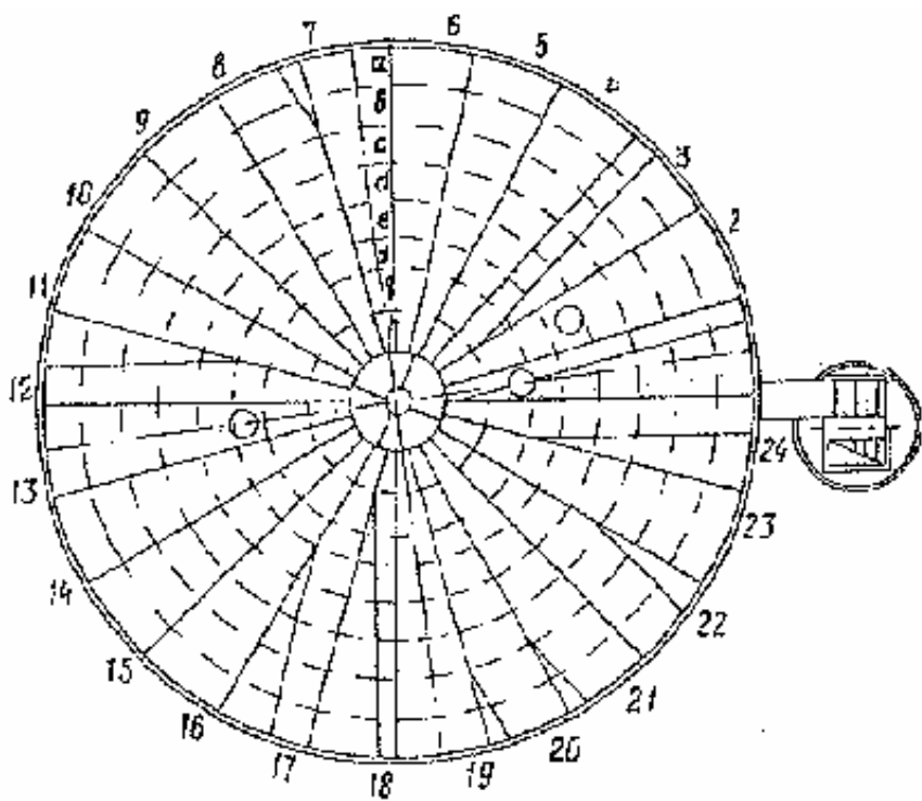
Рис. 3. Пример карты для обследования кровли бака
